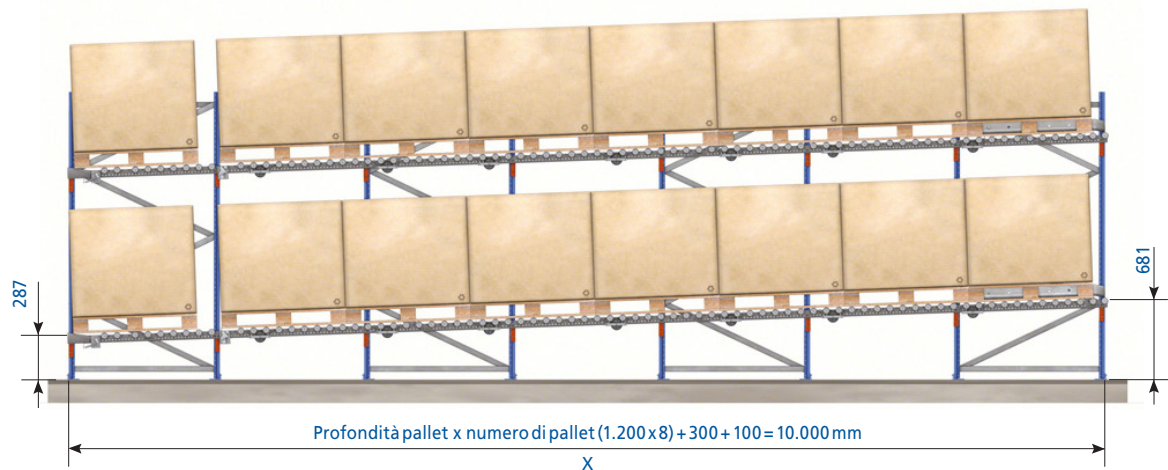
Figura 8. Esempio con arresto secondo pallet (pendenza del 4%)
