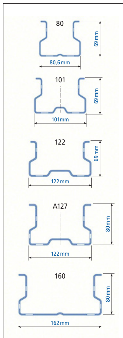
Figura 8. Montanti utilizzati.
