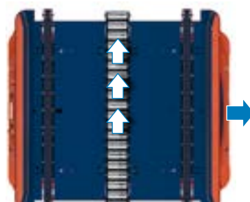
Trasmissione laterale dei carichi per europallet 1.200 x 800/1.000/1.200 mm.
